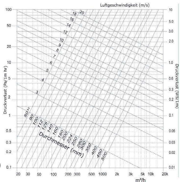
Druckverlust bei gerader Leitungsverlegung
